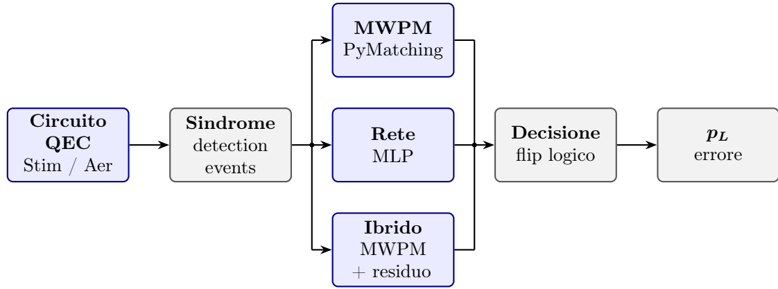
Figura 4.2: Flusso implementativo dei decoder: stessi detection event, regole decisionali differenti.
